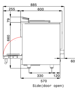
Boven aanzicht
