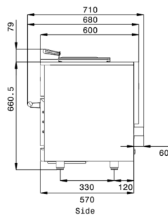
Zij aanzicht
