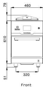
Front aanzicht
